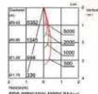
SDS-025K(15W 4000K,24deg)
